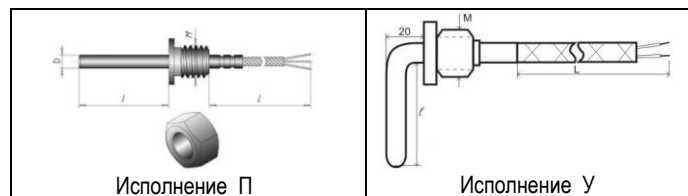
Рисунок 1 – Термопреобразователь сопротивления в конструктивном исполнении К4Р
