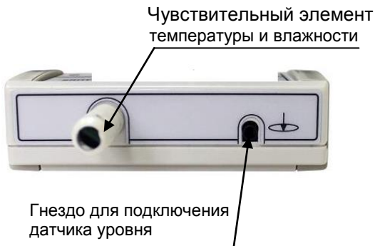
Рисунок 1 – Внешний вид датчика температуры и относительной влажности SRHT-GSM
